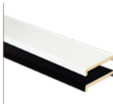
U-profile white or black - 240 x 0,45 x 6,6 cm
